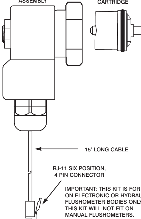
EL 297-A SOLENOID ASSEMBLY
